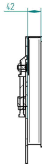
Schnitt A-A
