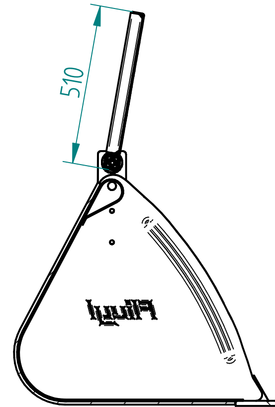
Schnitt A-A
