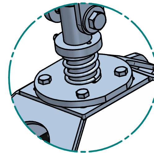
EINZELHEIT A
