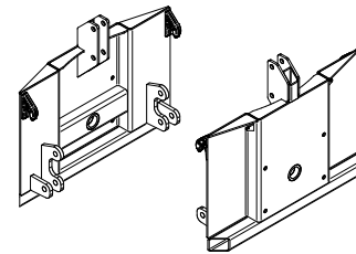
Aufnahmeadapter für Dreipunkt und Euronorm oder Hof-, Rad- oder Teleskopladeraufnahme
