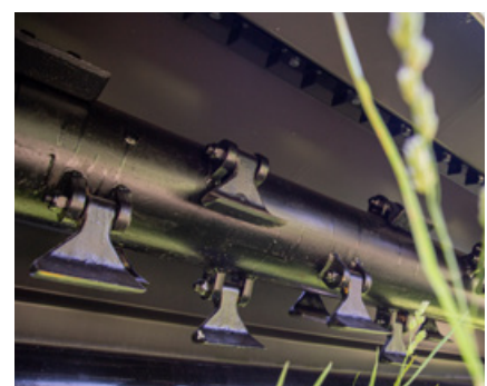
Abb.: extrem verschleißfeste Hammerschlegel
