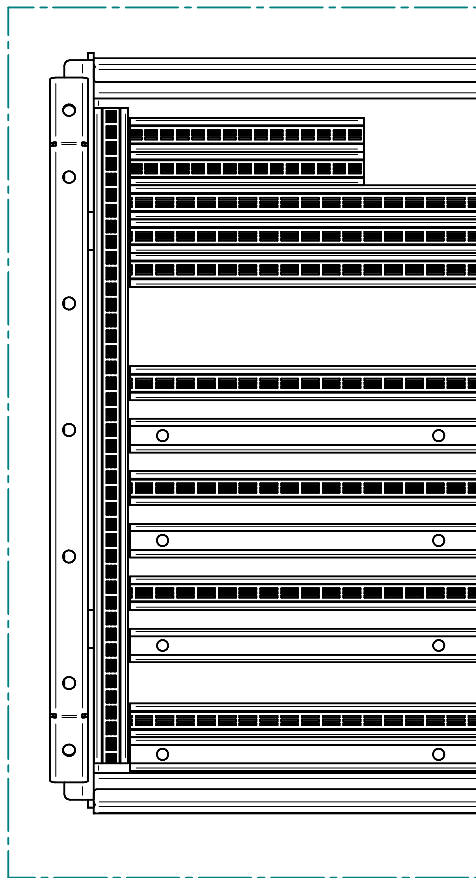
Einzelheit A
