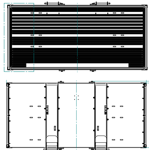
Abb. 22 Reihen aus robusten Kehrborsten
