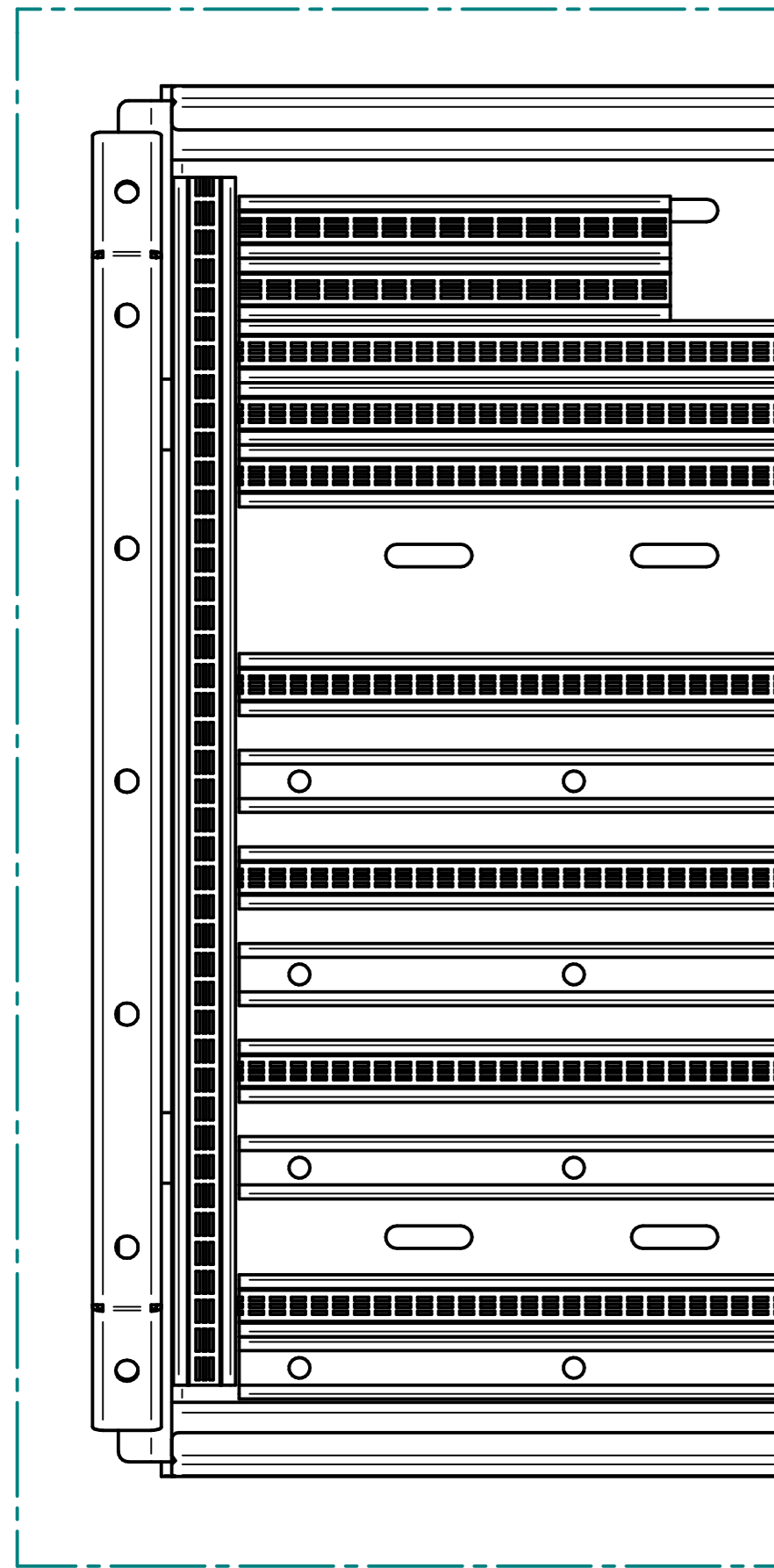
Einzelheit A
