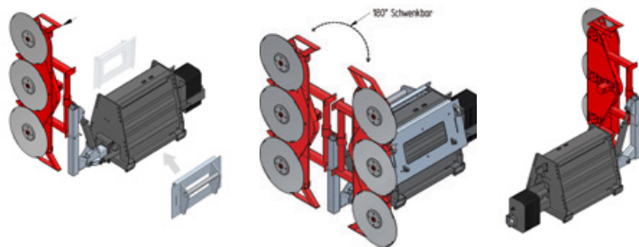
Abb.: Verwendung bei Teleskoplader mit Linksanbau
