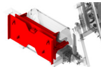
Überlastsicherung: Bei zu hohem Anpressdruck neigt sich der Kopf nach hinten zum Schutz vor Blockieren.
